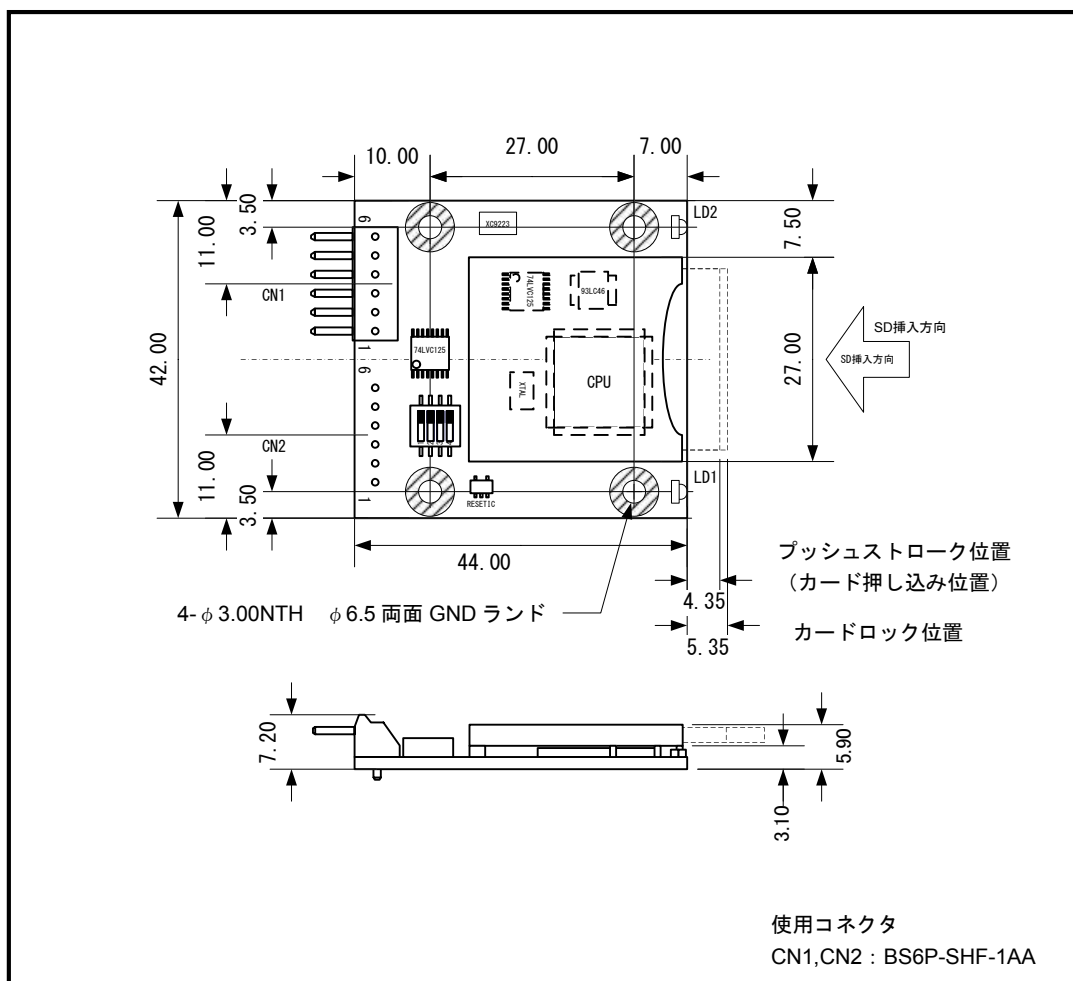
Fig 2.6-1 外形寸法図
