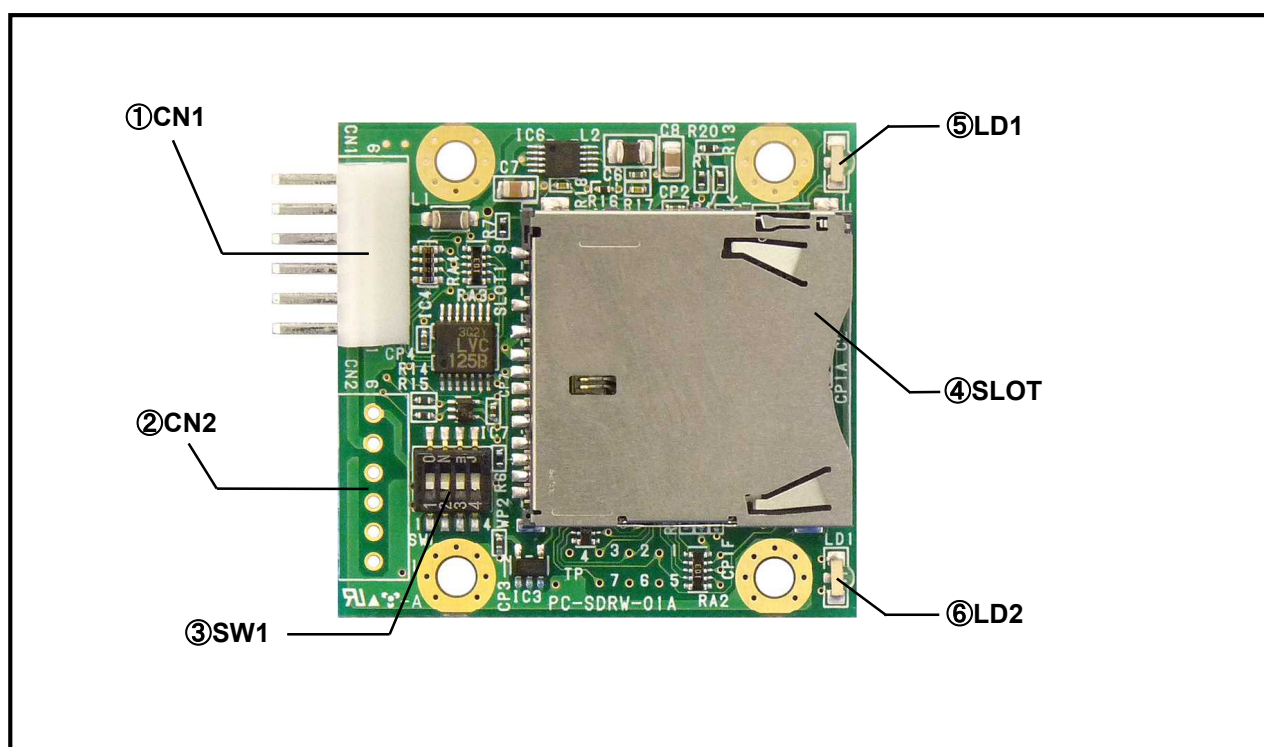
Fig 2.5-1 外形図
