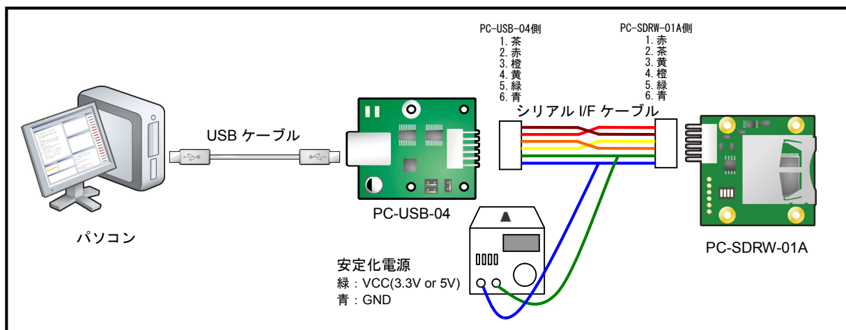
Fig 5.3-1 パソコンと PC-SDRW-01A の接続例
