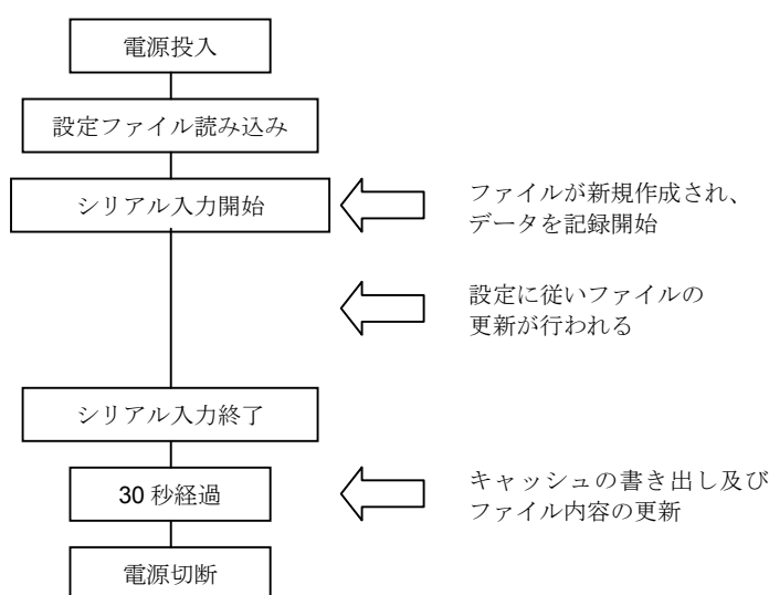
Fig 4.4-1 自動ロギングモードの基本動作例
