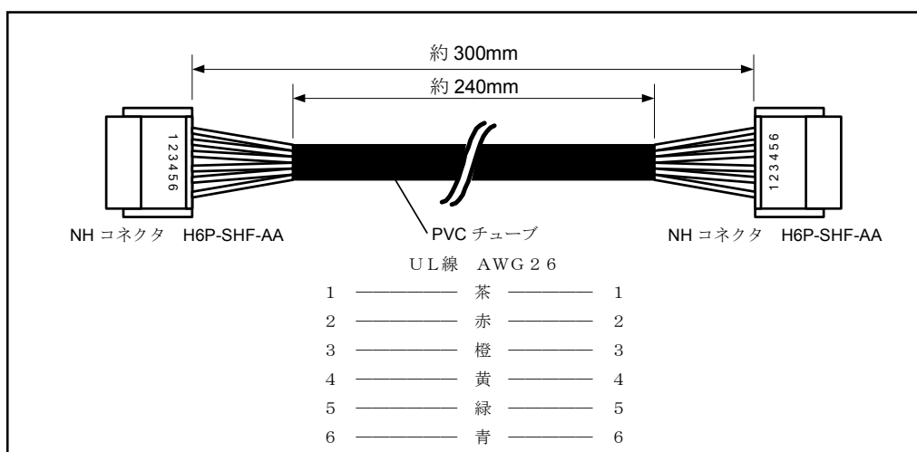
Fig 2.6-2 シリアル I/F ケーブル寸法図
