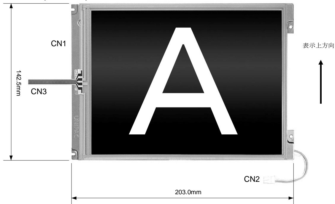
Fig 2.2.1 LCD パネル(B084SN03V.2)外形図
