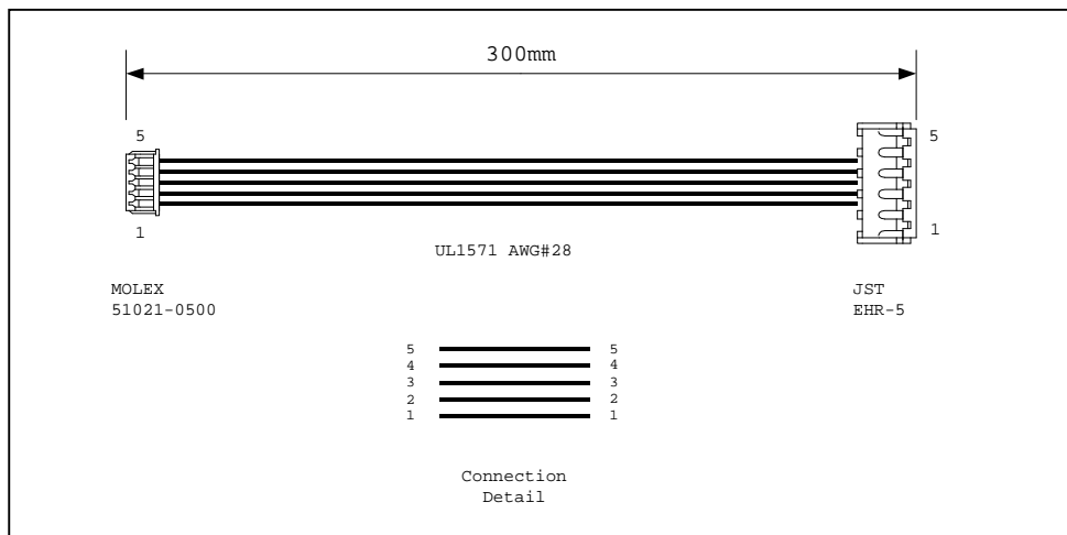
Fig 2.2.5 インバータ用ケーブル
