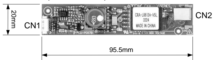
Fig 2.2.2 インバータ(CXA-L0612A-VSL)外形図
