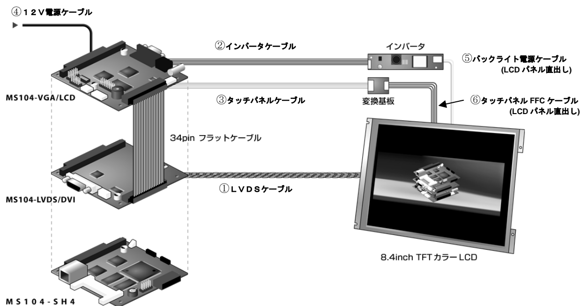
Fig 3.4.2 MS104シリーズとの接続図
