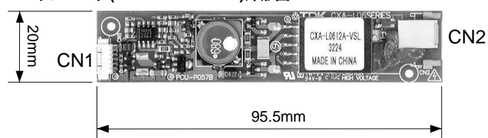
Fig 2.2.2 インバータ(CXA-L0612A-VSL)外形図
