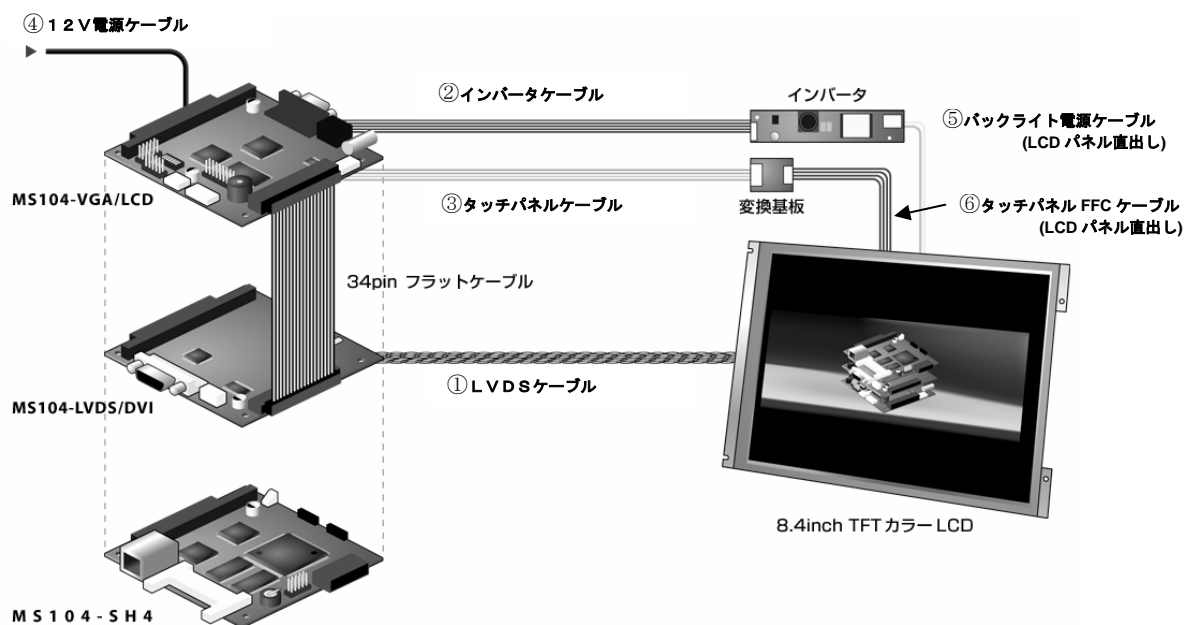
Fig 3.4.2 MS104シリーズとの接続図
