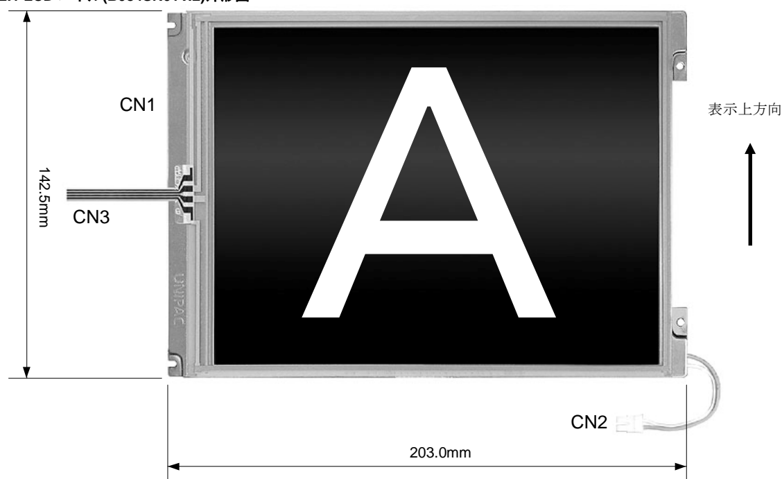
Fig 2.2.1 LCD パネル(B084SN01V.2)外形図
