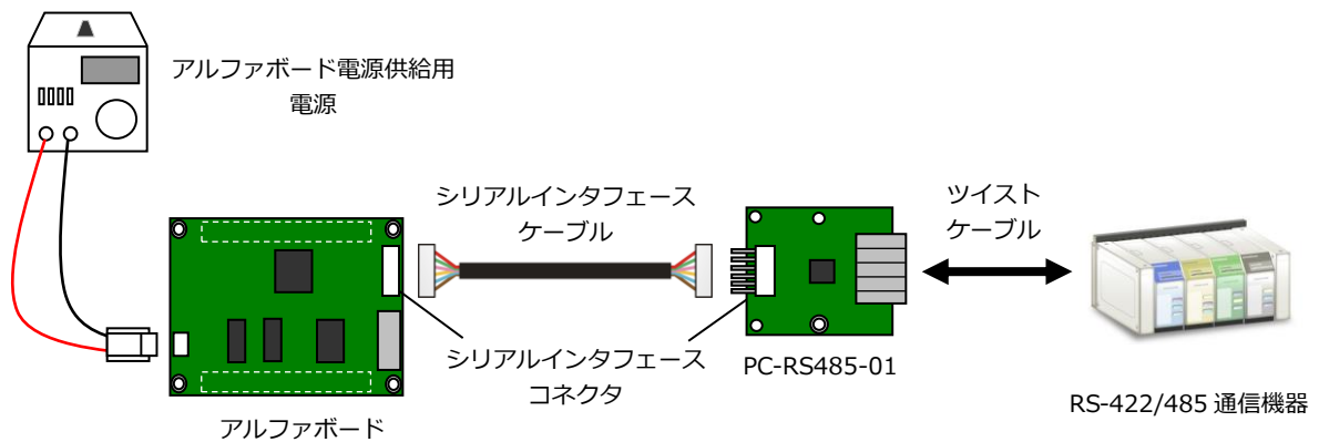
Fig 3.2-1 PC-RS485-01 とアルファボードとの接続例
