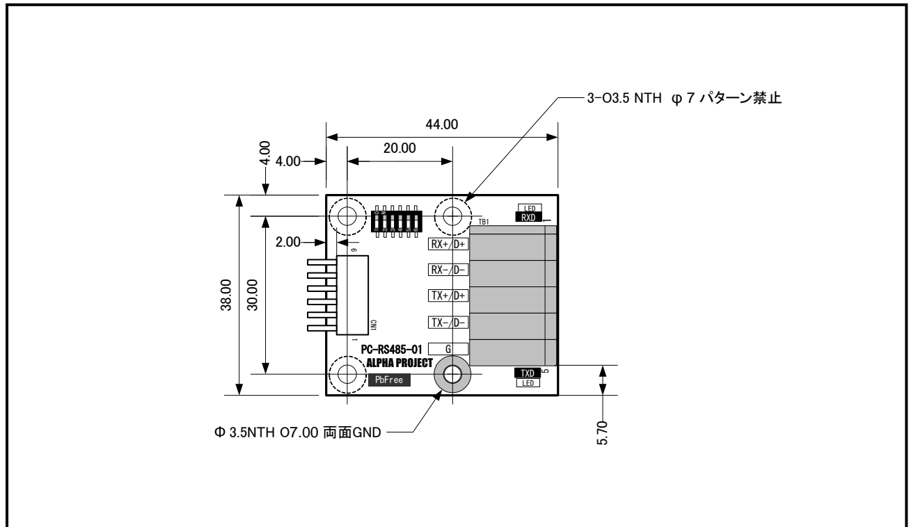
Fig 3.1-1 PC-RS485-01 外形寸法図
