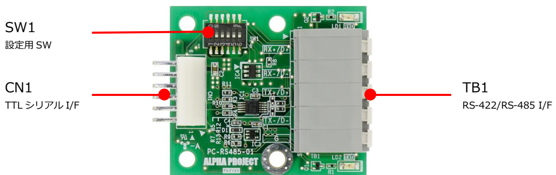
Fig 1.7-1 外形図
