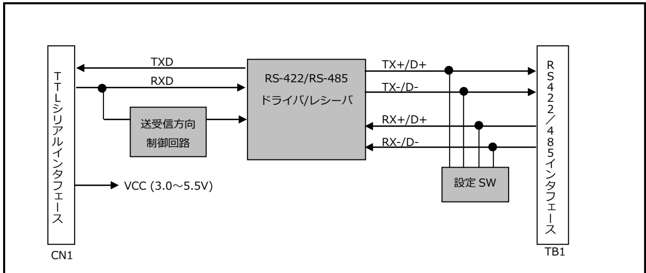
Fig 1.6-1 PC-RS485-01 構成ブロック図
