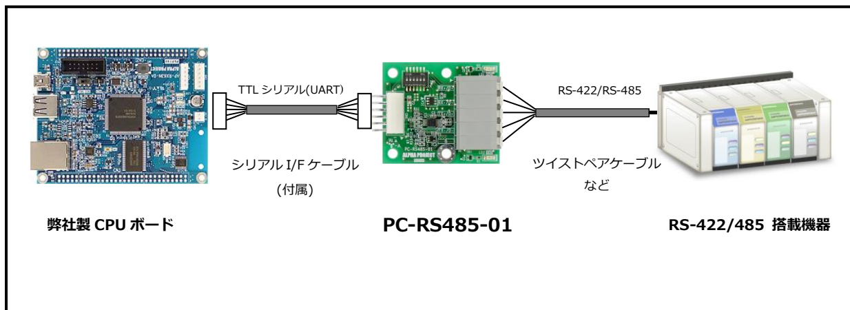
Fig 1.3-1 PC-RS485-01 接続イメージ
