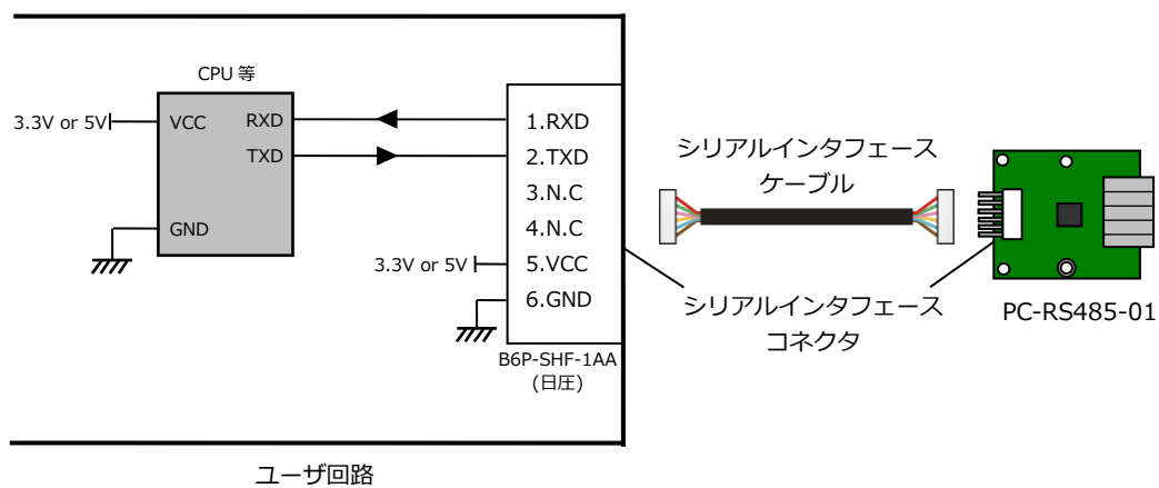
Fig 3.2-2 PC-RS485-01 とユーザ回路との接続例
