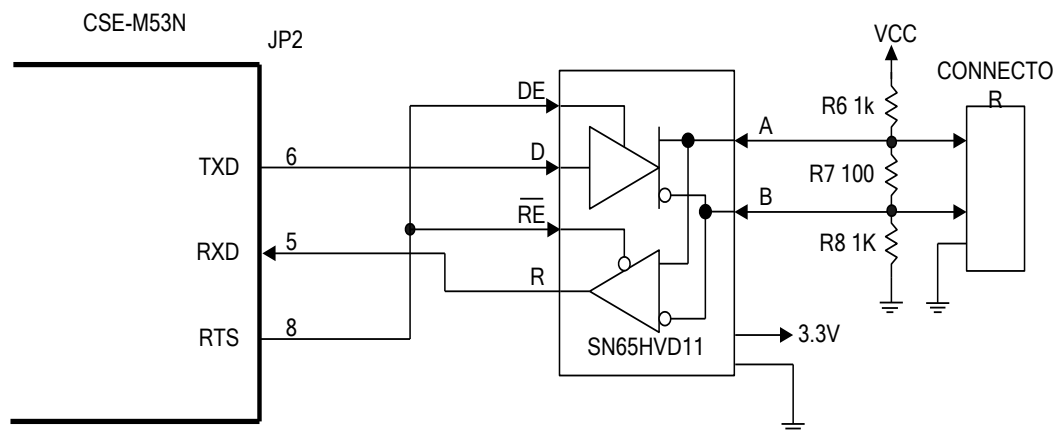
Fig 8.1-5 RS485 ドライバの接続
