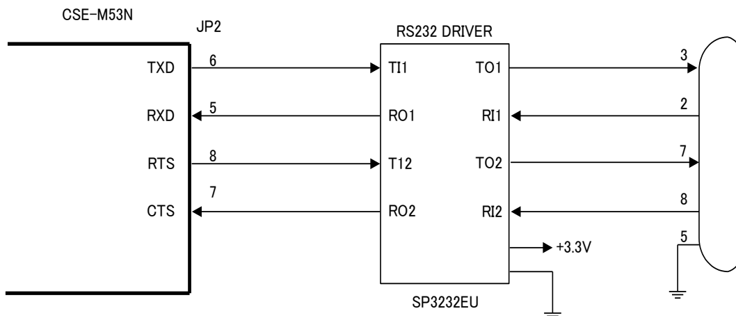
Fig 8.1-4 RS232 ドライバの接続
