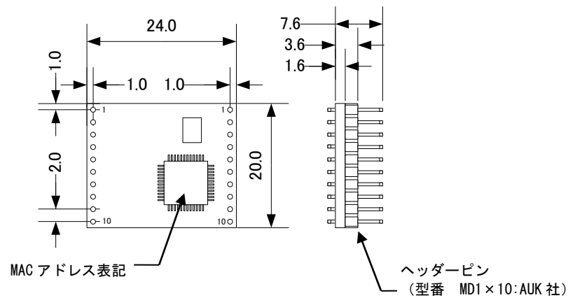
Fig 1.6-1 外形寸法図
