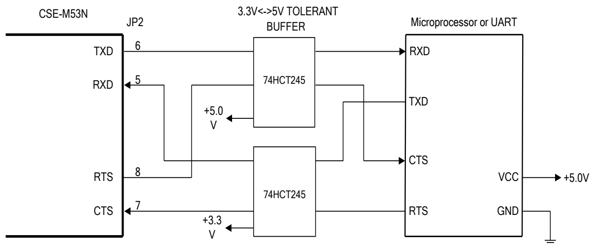
Fig 8.1-3 5.0V マイコンの接続
