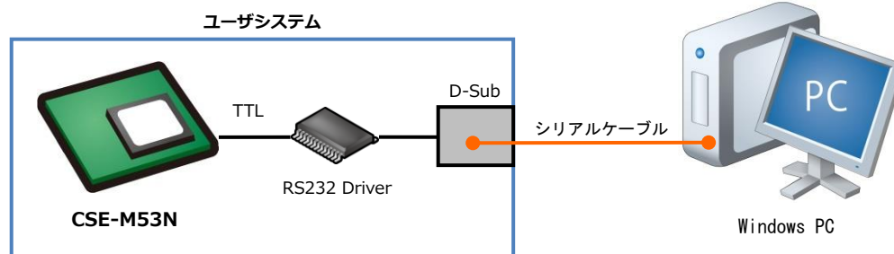
Fig 3.2-6 ezManager シリアルインタフェースからの設定変更
