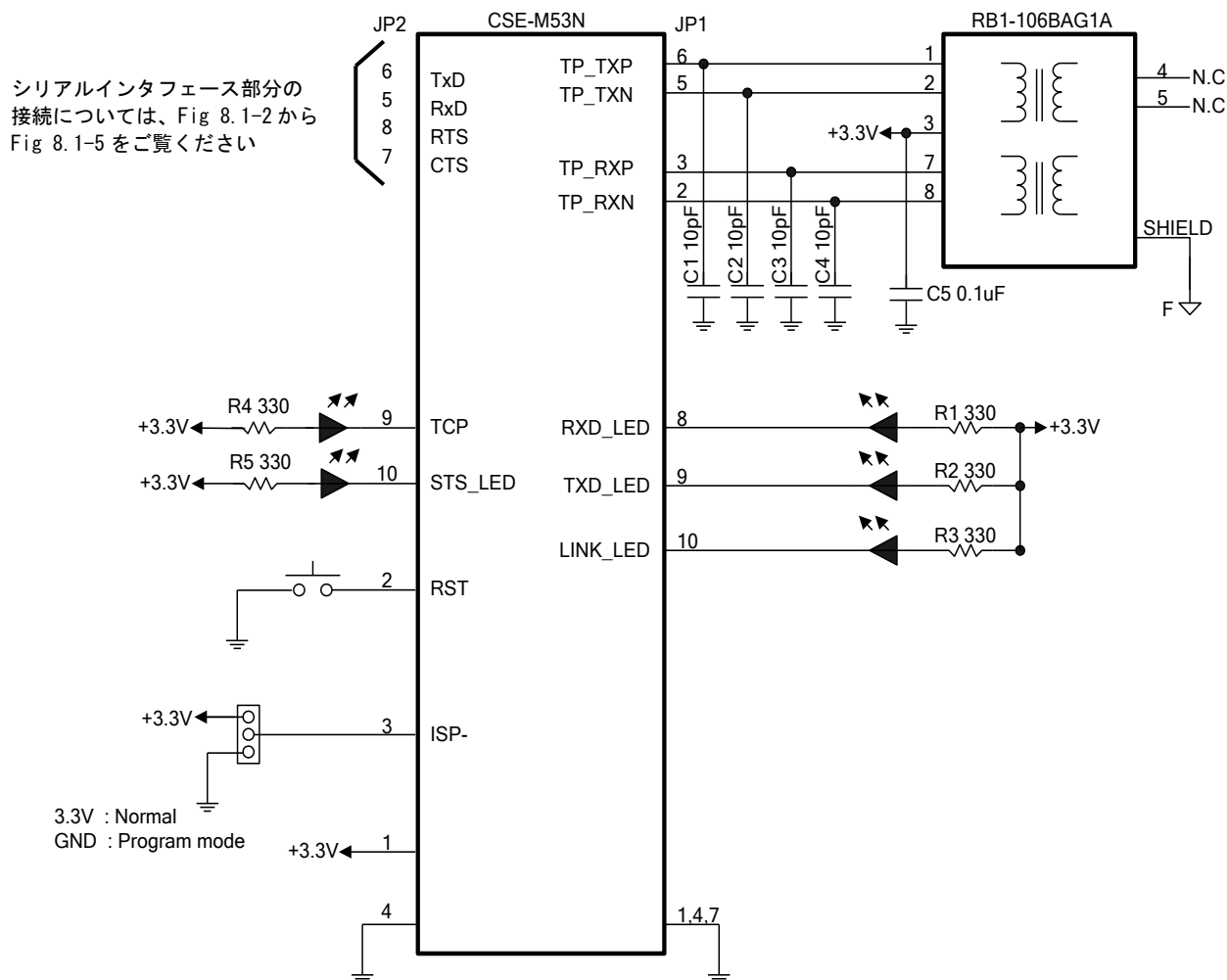
Fig 8.1-1 CSE-M53N 接続図
