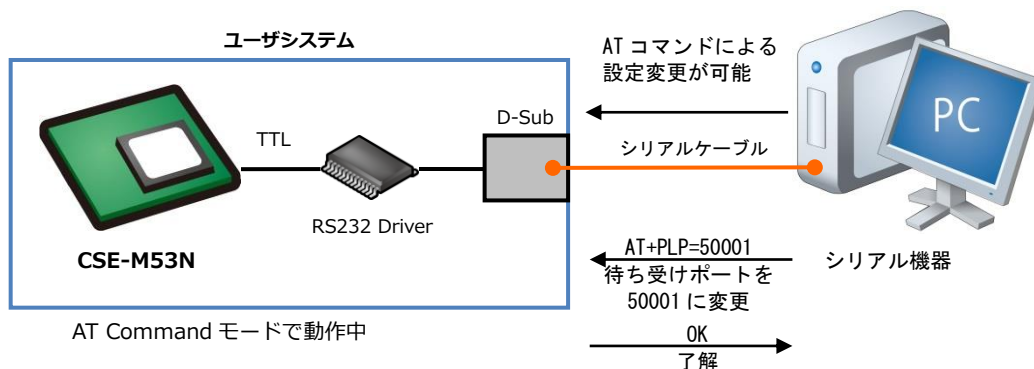
Fig 3.3-1 AT コマンドによる設定変更
