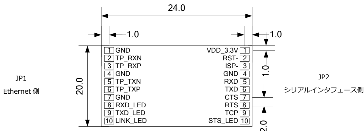
Fig 1.6-3 コネクタピン配置
