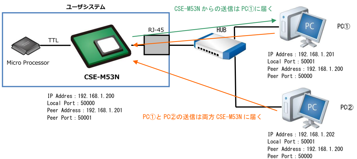
Fig 5.7-4 ユニキャスト通信構成例 2
