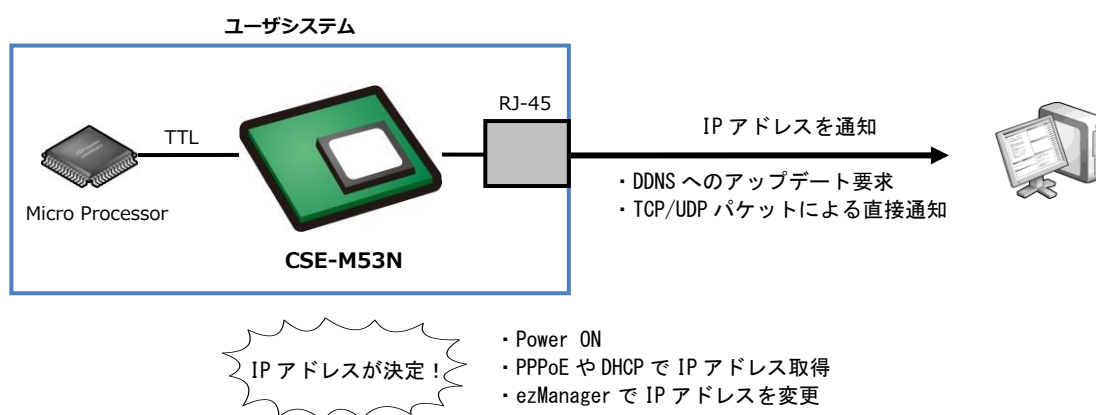
Fig 6.3-1 IP アドレス通知機能 (Notify IP Change)
