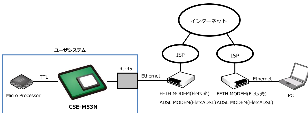
Fig 1.4-5 ネットワーク接続例③
