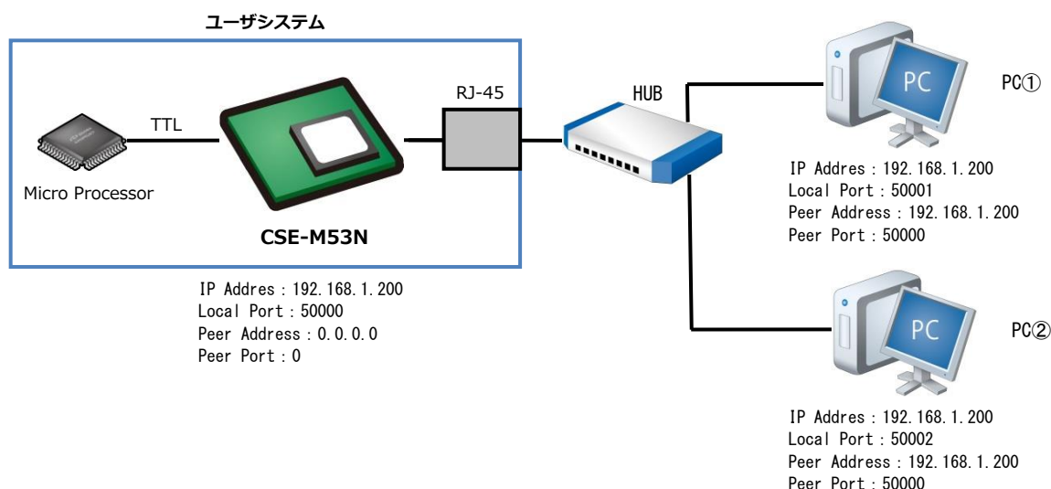
Fig 5.7-7 U2S エコー通信構成例
