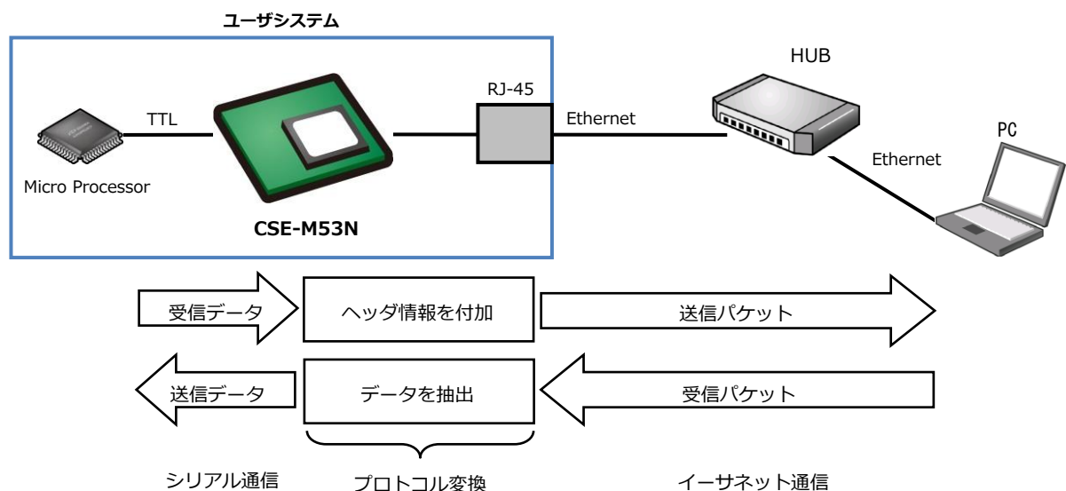
Fig 1.3-1 プロトコル変換の仕組み
