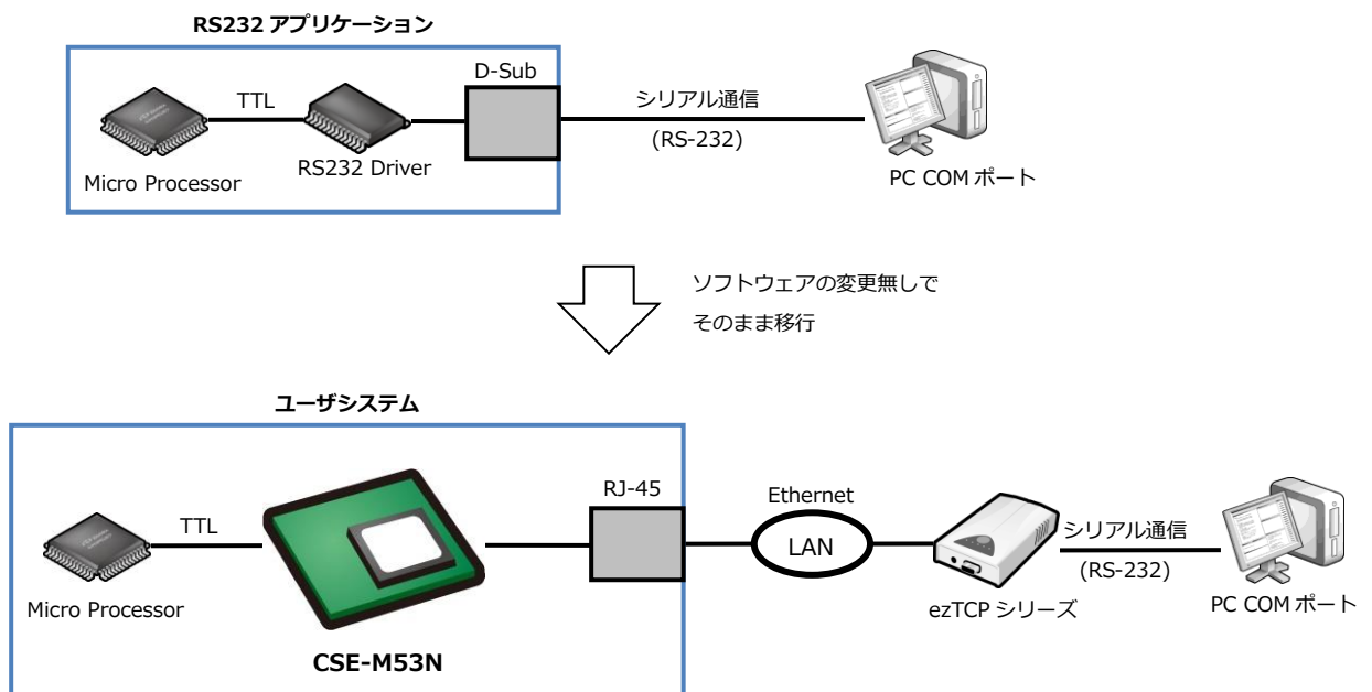
Fig 1.4-2 既存の RS232 ネットワークをイーサネットへ接続
