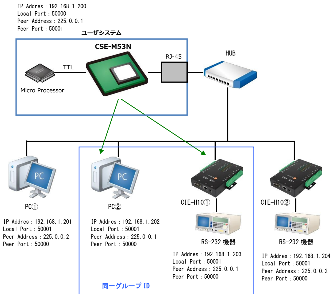
Fig 5.7-6 マルチキャスト通信構成例
