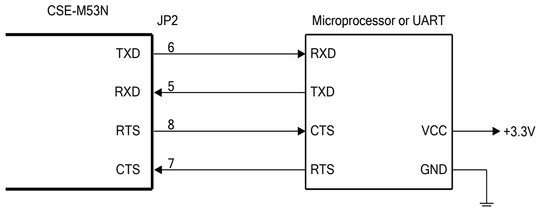
Fig 8.1-2 3.3V マイコンの接続
