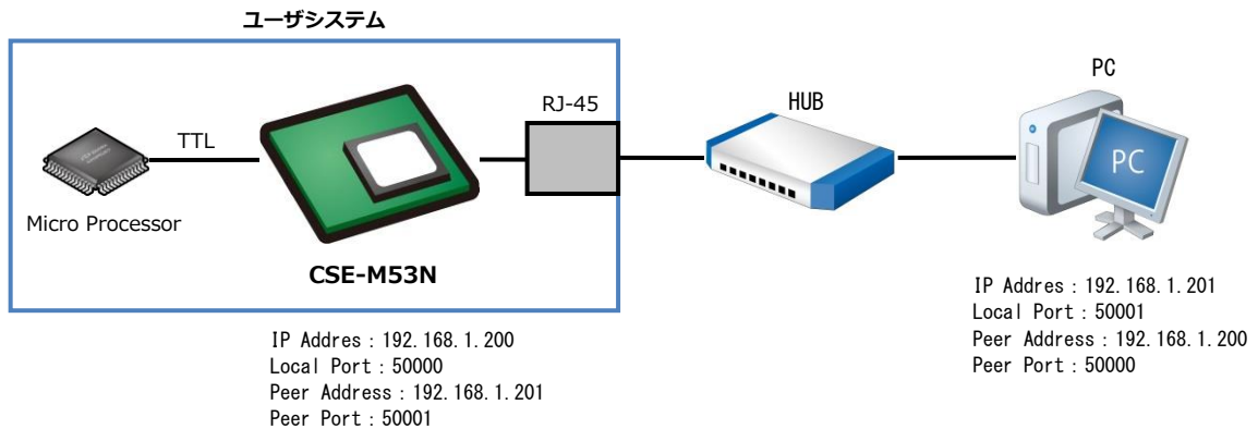
Fig 5.7-3 ユニキャスト通信構成例 1
