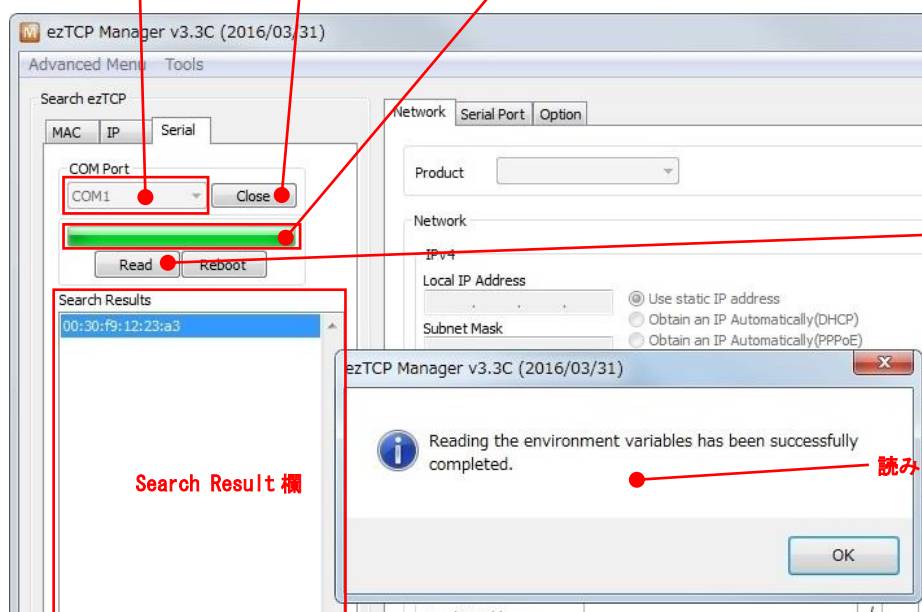
Fig 3.2-8 ezManager シリアルインタフェースからの設定値読み出し
