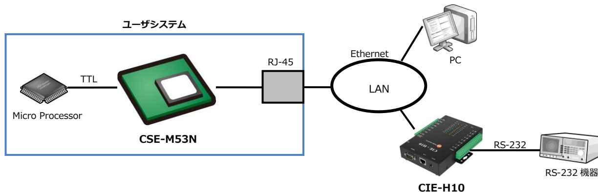
Fig 1.4-3 ネットワーク接続例①
