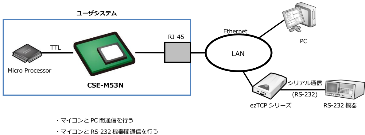
Fig 1.4-1 基本的な接続例
