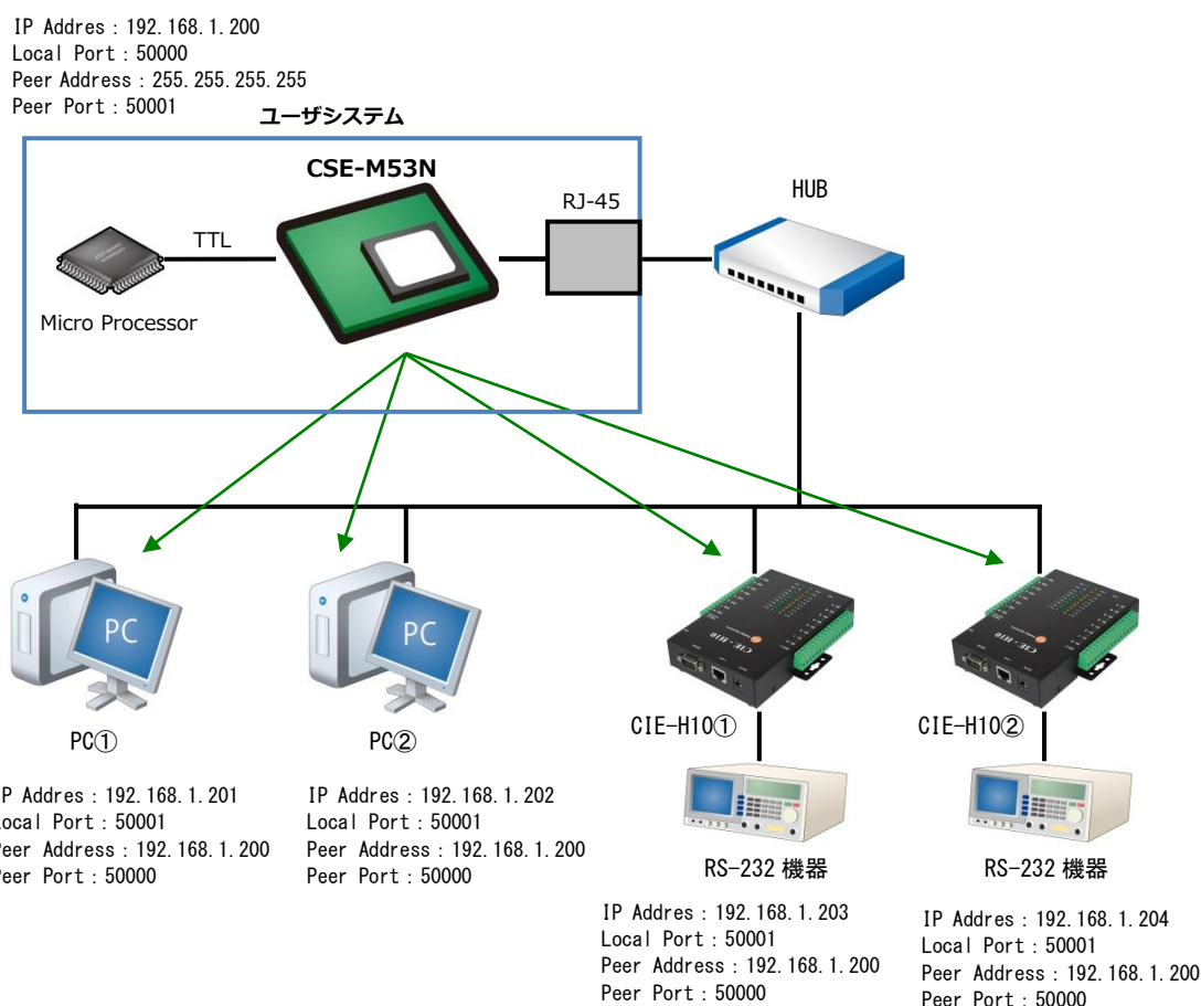
Fig 5.7-5 ブロードキャスト通信構成例
