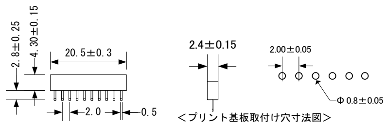
Fig 1.6-2 レセプタクル (付属) (型番 SD1-10:AUK 社)
