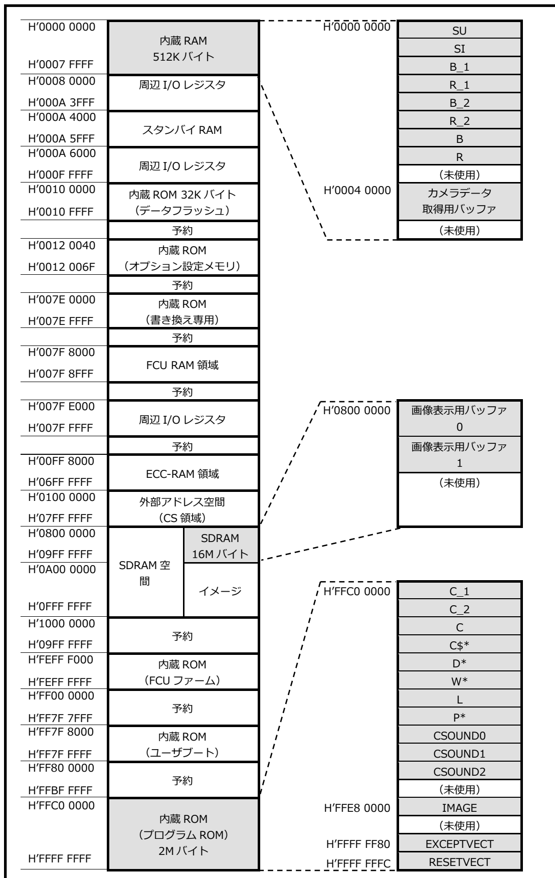
Fig 3.2-1 LCD-KIT + VS-CAM-01 サンプルプログラム(AP-RX71M-0A) メモリマップ
