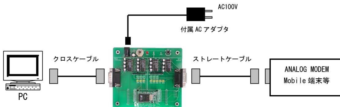
図2. 1-1 評価ボードの接続例
