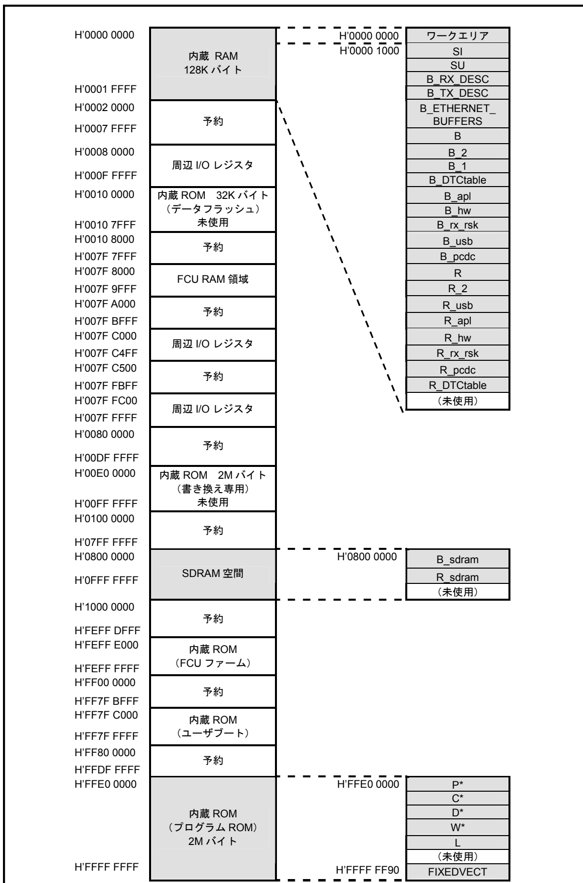
Fig 3.2-1 ネットワーク通信 + USB ファンクションサンプルプログラムメモリマップ
