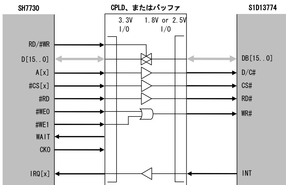
Fig 2.2-1 接続例
